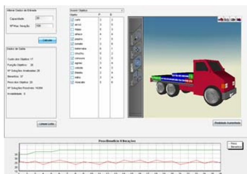
Figura 4 Interface do sistema.
