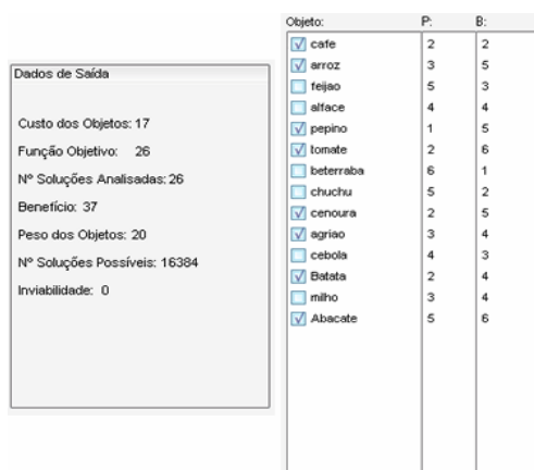
Figura 2 Dados de saída.
